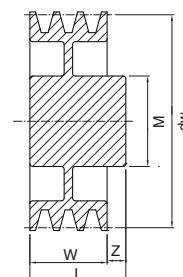
4 4A (z otworami zmniejszającymi wagę)
