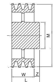
8 (3 żebra) 8A (6 żeber)
